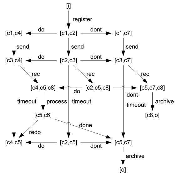
FIGURE 7. The OG of system S
